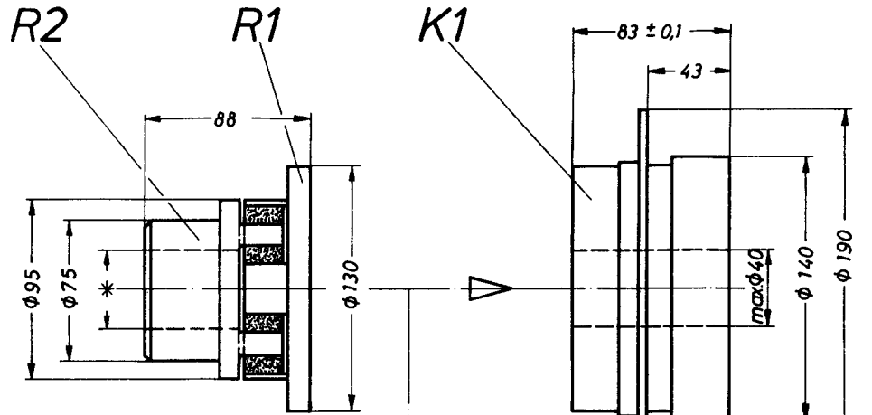
Ausführung „A“ 42 CF * Bohrung von \phi 14 bis max. \phi 42
