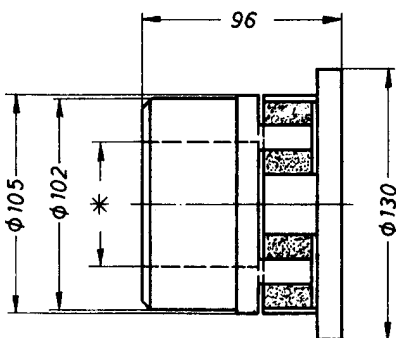
Ausführung „D“ 48/60 * Bohrung von \phi 48 bis max. \phi 60
