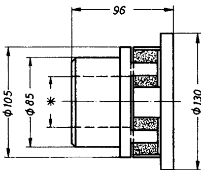
Ausführung „C“ 48 CF * Bohrung von \phi 15 bis max. \phi 48
