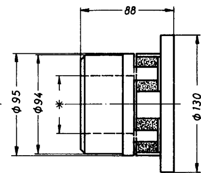
Ausführung „B“ 42/55 * Bohrung von \phi 42 bis max. \phi 55
